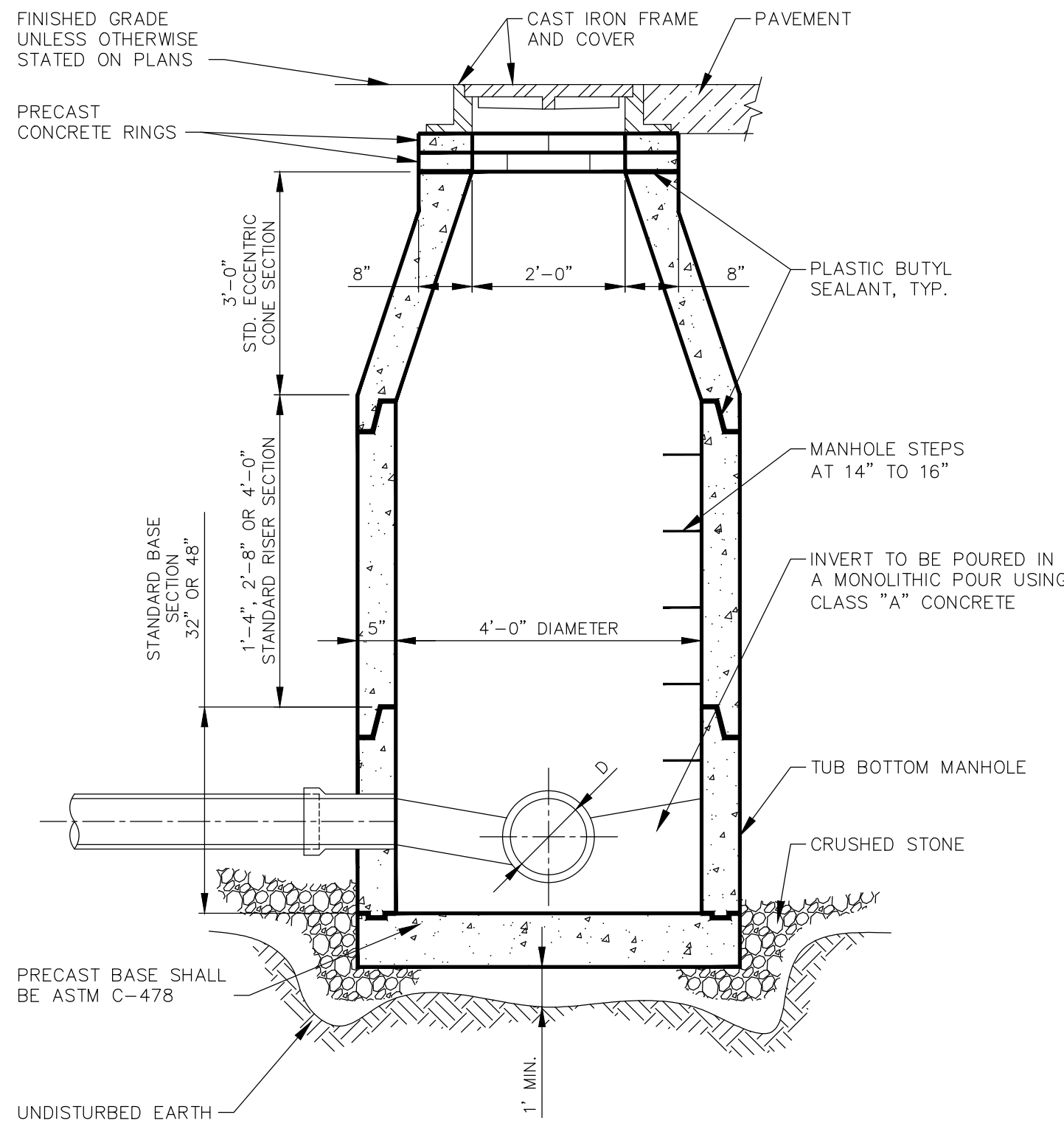
STANDARD PRECAST MANHOLE N.T.S.
