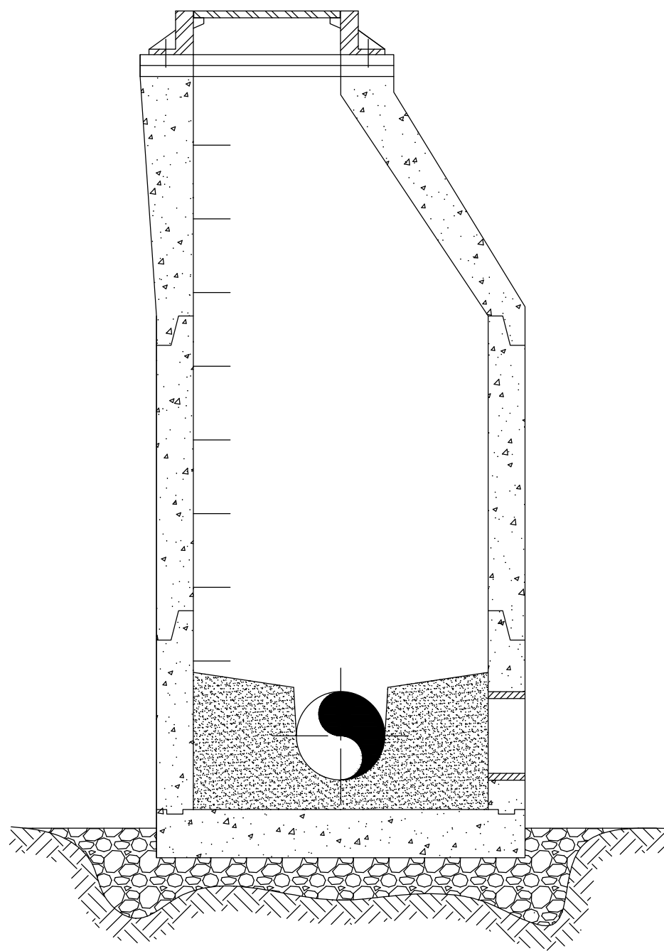
STANDARD MANHOLE FOR SEWERS N.T.S.
